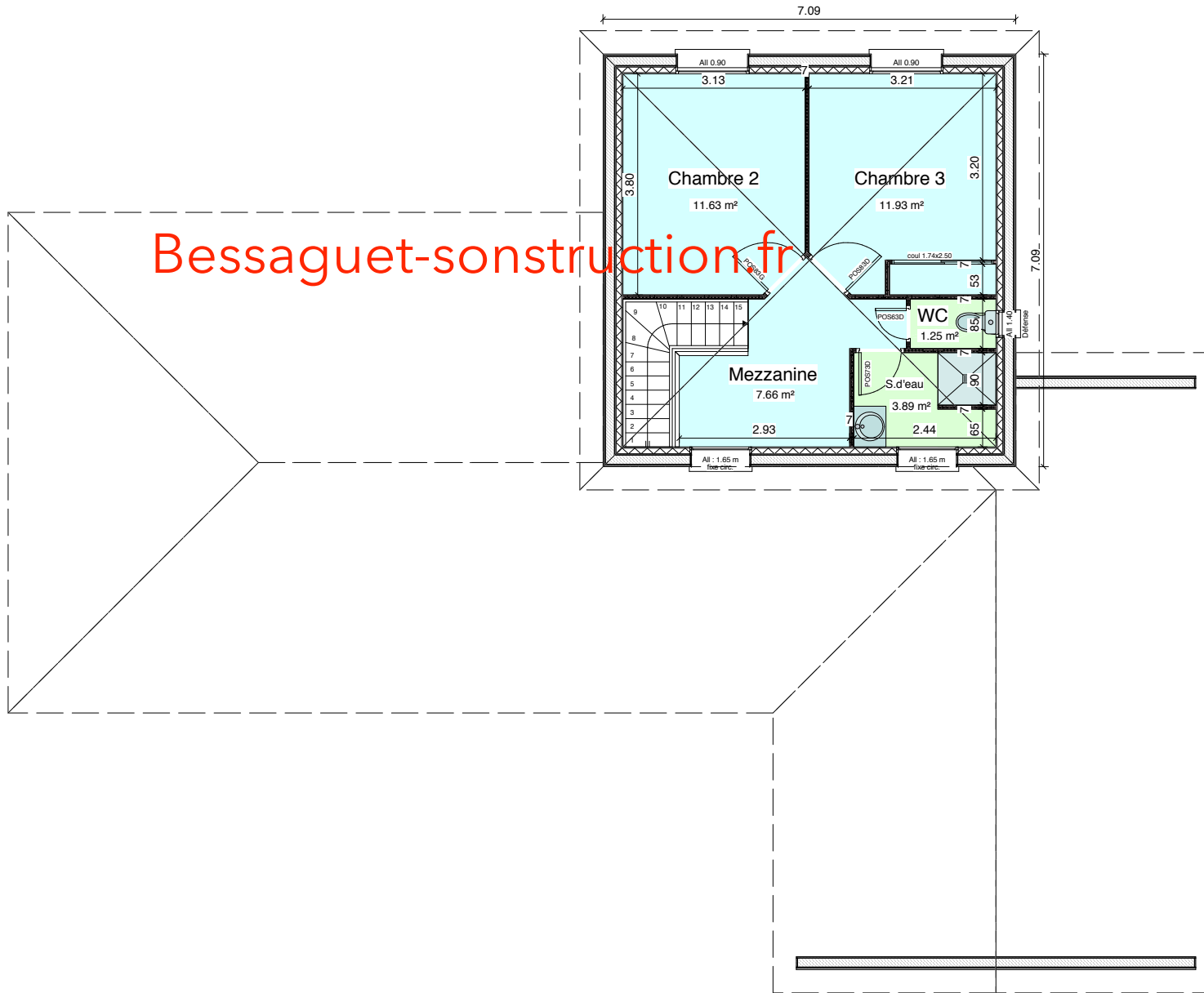
ETAGE 36,36 m 2
